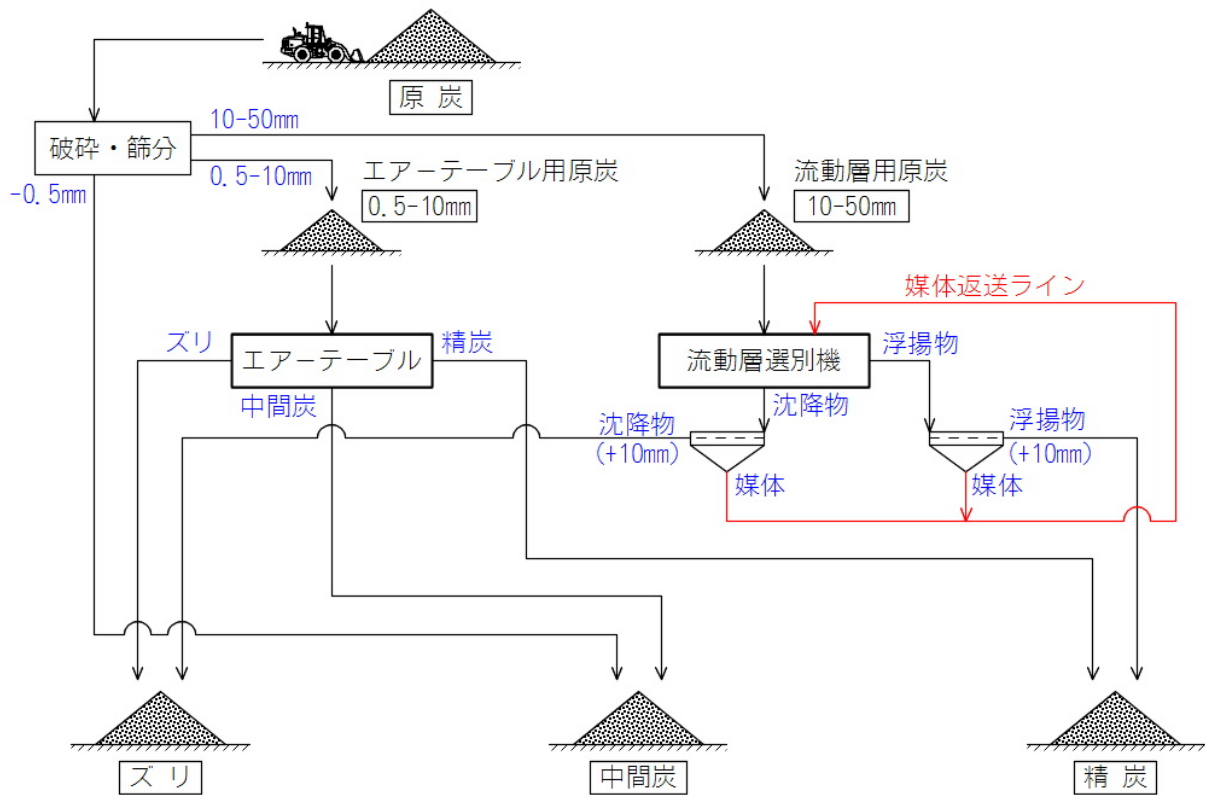
【乾式選炭システムフロー図】
